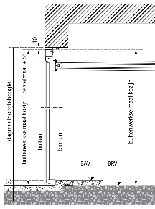
Verticale doorsnede
