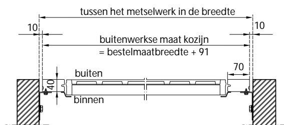
Horizontale doorsnede
