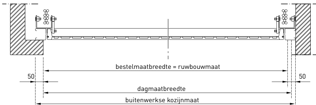
horizontale doorsnede
