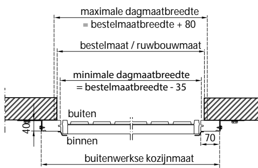
Horizontale doorsnede
